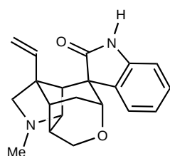
1: gelsemine
