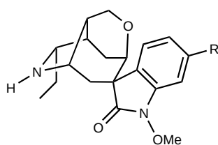
2: gelsedine, R = H 3: gelsemicine, R = OMe
